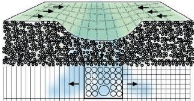
Mulden-Rigolen-Element (BSU Hamburg 2006: 34)
